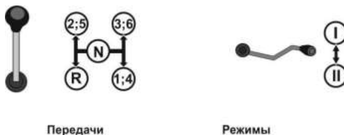
Рисунок 3.9. Переключение передач и режимов Трактора малогабаритного РУСИЧ модель Т-12 (12л.с.)
